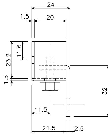
D30 ステン壁付ソケット (13T36)
