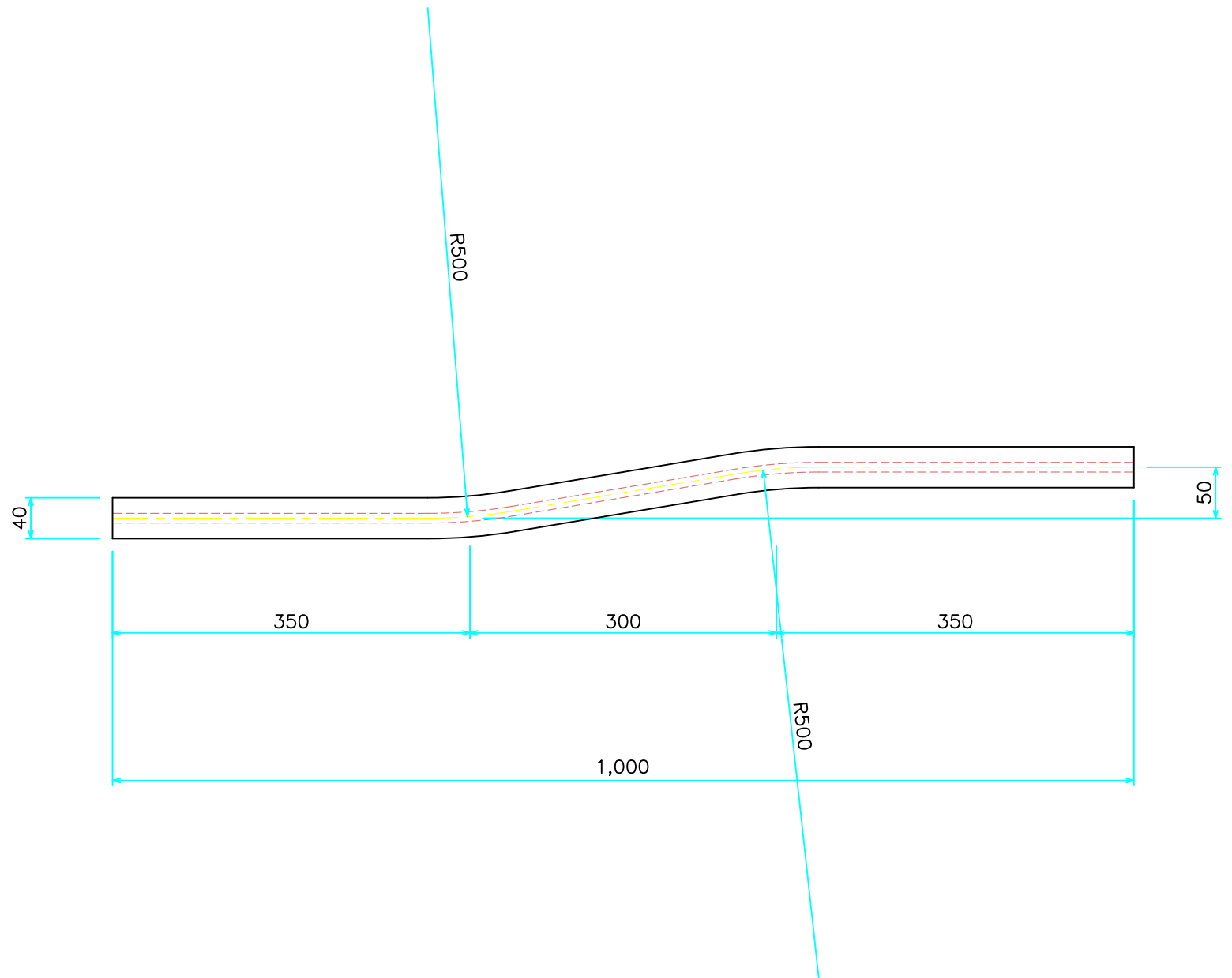
D40交又レール・アルミ (15L07-AS)
