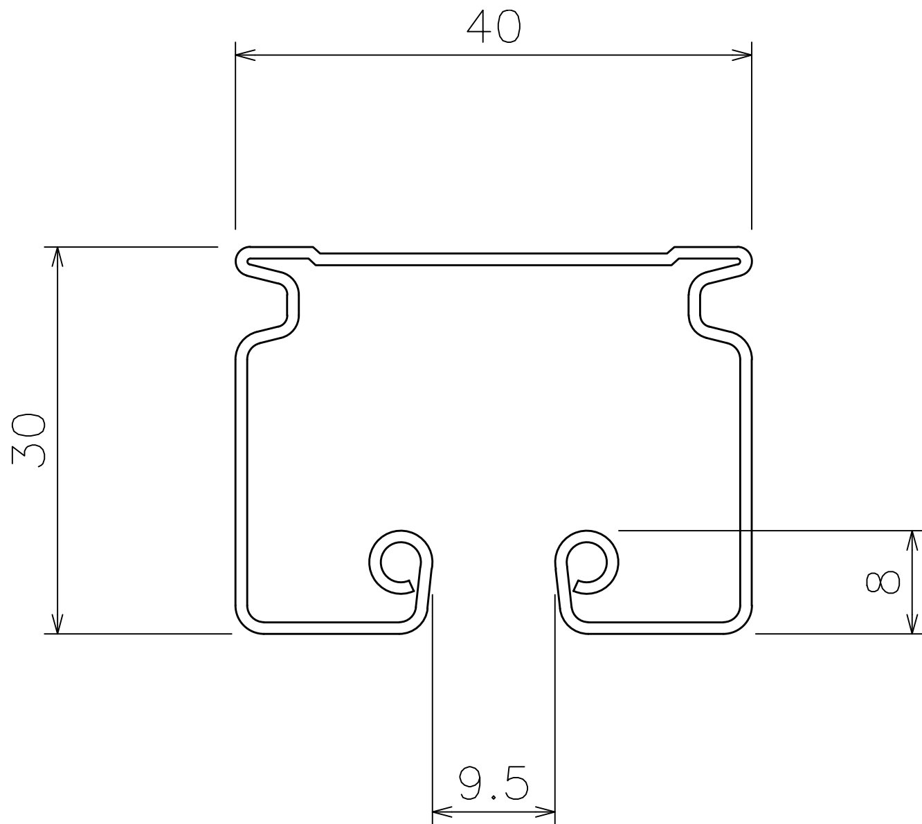
D40 ステンレスレール ( 25L ※※ -SU )
