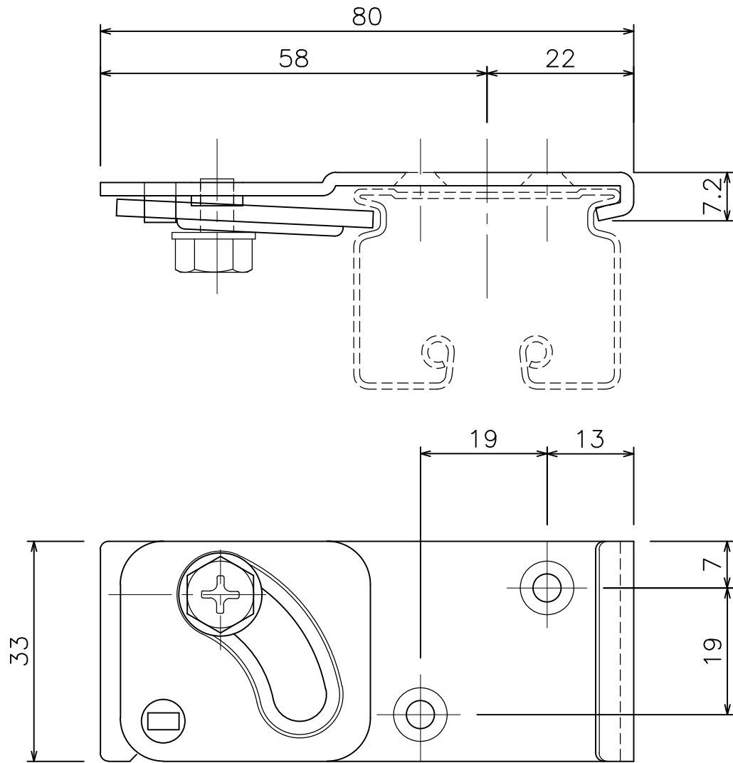
D40 ステン天井Sブラケット (25T51)
