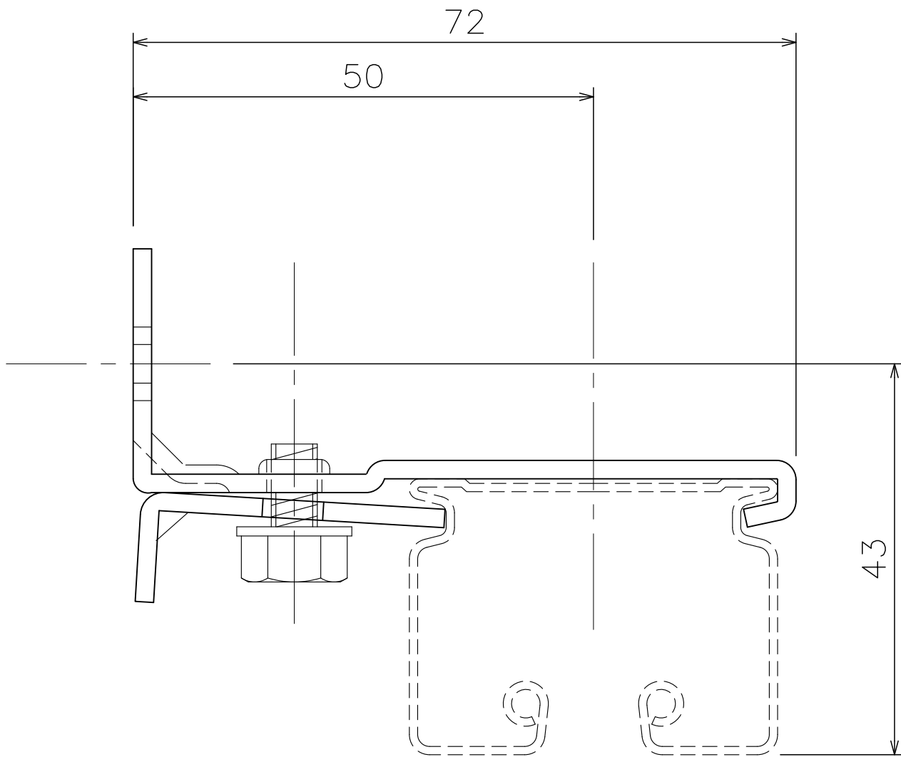
D40 ステンSブラケット (25T 41)
