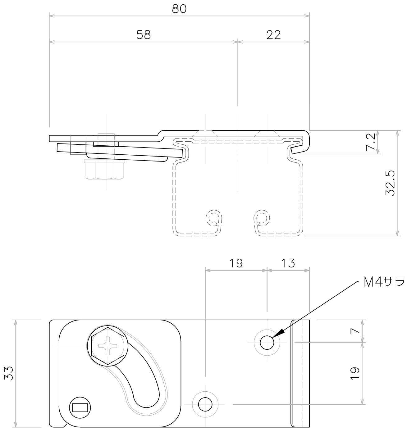
D40 天井Sブラケット (15T51)
