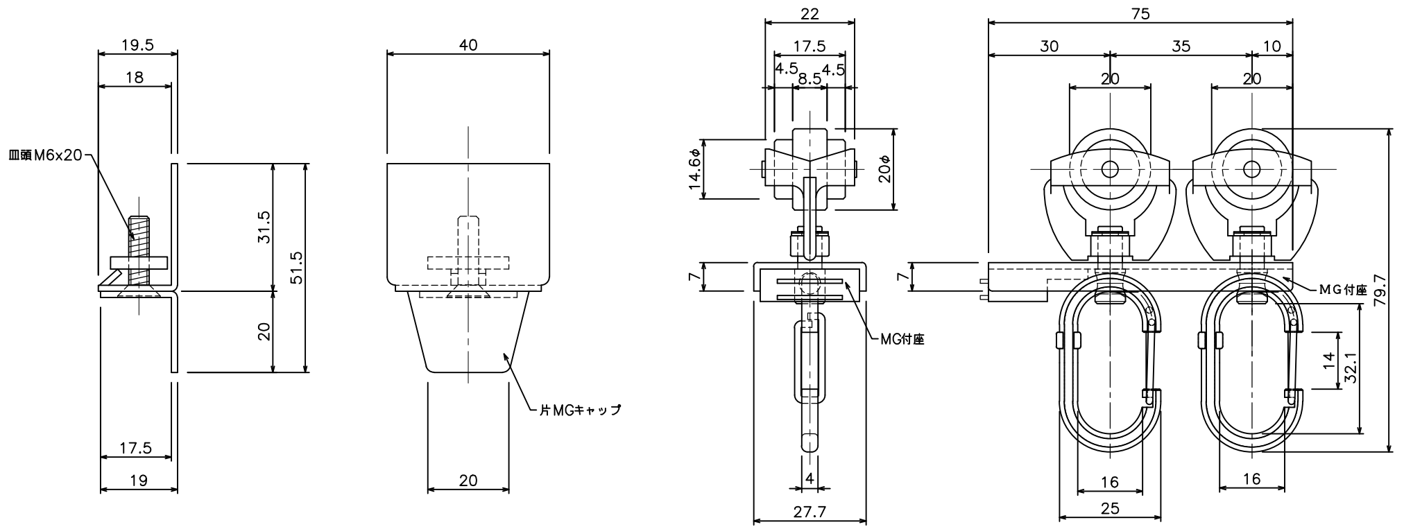
D40片マグネットランナー(片開)ワンタッチランナー S (15Y34)
