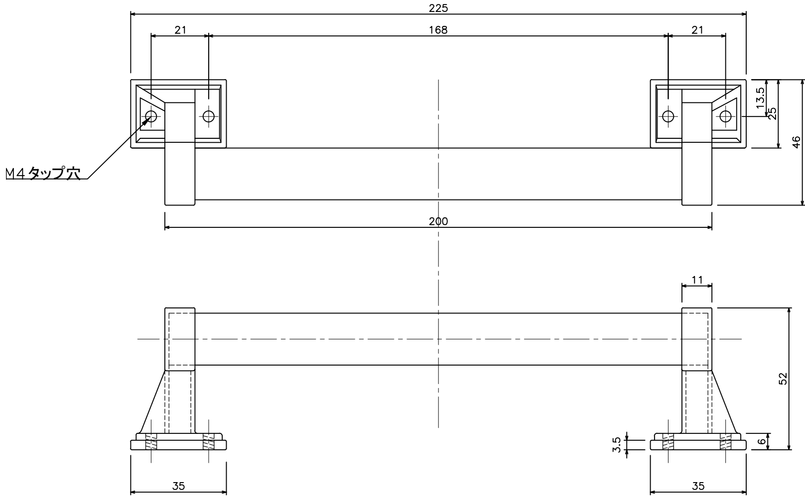
間仕切 アルミパイプ取手 (90T67)
