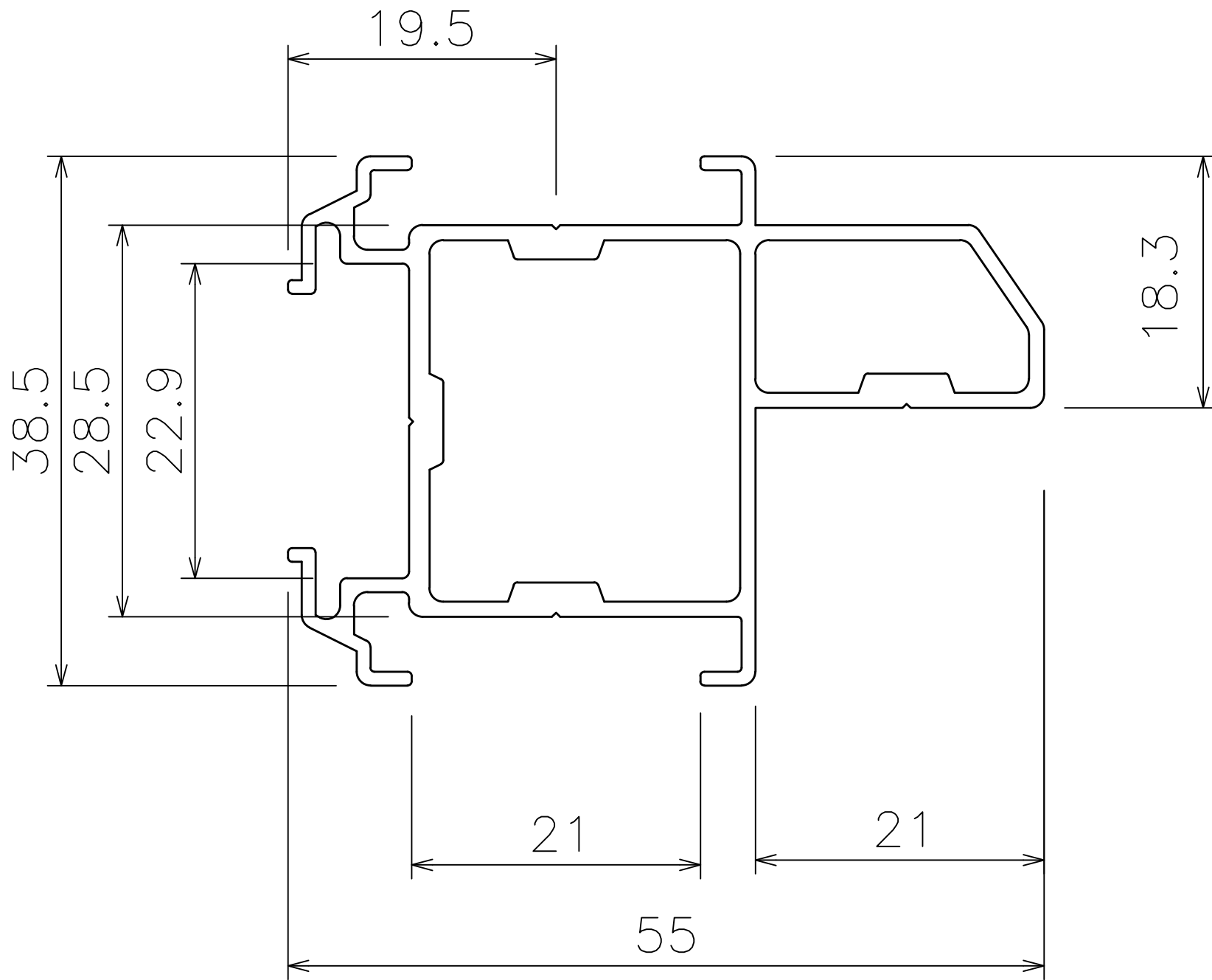
間仕切 サイドポール 押えバー (90S***)
